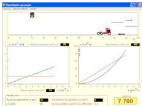
4. Διαγραμματική μελέτη μιας τυπικής προσπέρασης ενός φορτηγού.
