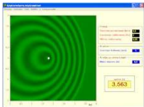
24. Φαινόμενο Doppler πάνω στην επιφάνεια υγρού, με ομαλά κινούμενη πηγή ή ακίνητο μέσο ή ακίνητη πηγή σε ομαλά κινούμενο μέσο.
