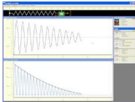
5. Φθίνουσες μηχανικές ταλαντώσεις, επάνω σε οριζόντιο επίπεδο, με σταθερή τριβή ολίσθησης
