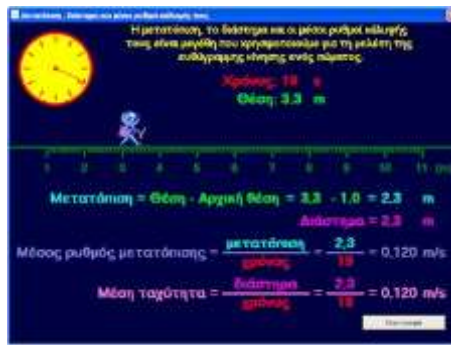
2. Μετατόπιση, διάστημα και οι μέσοι ρυθμοί κάλυψής τους
