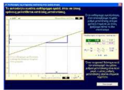
3. Διαγραμματικός υπολογισμός της ταχύτητας στην ομαλή κίνηση ως κλίση στο διάγραμμα θέσης με το χρόνο.
