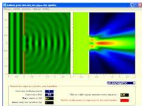
19. Διάδοση κυμάτων μέσα από οπές ή γύρω από εμπόδια στην επιφάνεια υγρών (περίθλαση)
