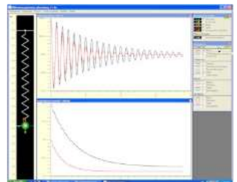
6. Φθίνουσες μηχανικές ταλαντώσεις, με τριβές της μορφής F = -bv .
