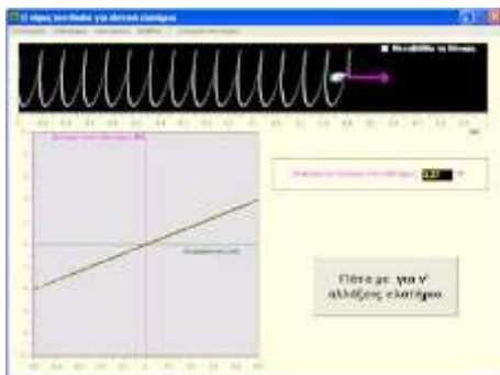
9. Ο νόμος του Hooke σε ιδανικά ελατήρια και σύγκριση ελατηρίων
