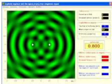
16. Συμβολή αρμονικών κυμάτων στην επιφάνεια υγρού από δύο πηγές.
