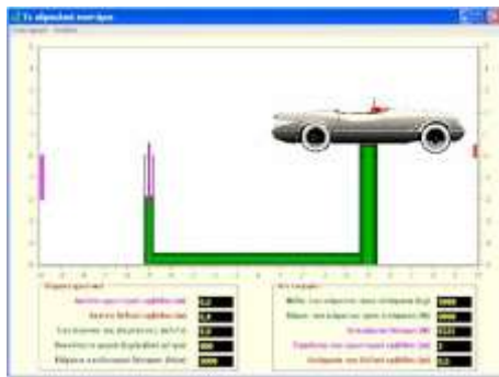
1. Το υδραυλικό πιεστήριο του Pascal
