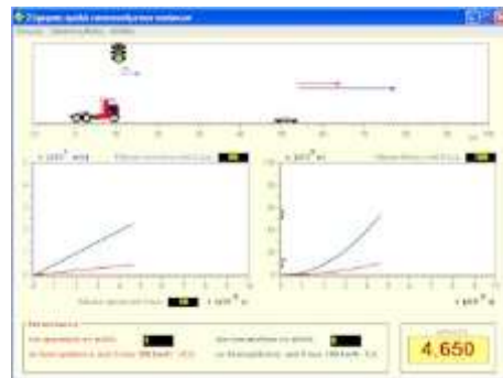
3. Σύγκριση ομαλά επιταχυνόμενων κινήσεων
