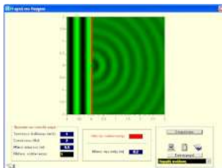
20. Η αρχή του Huygens
